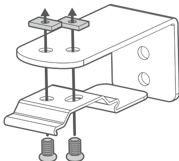
Väggmontering
